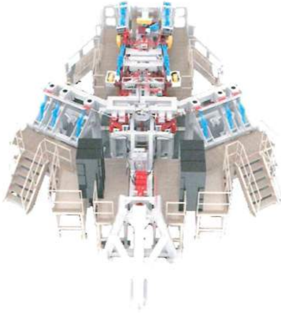
Şekil 55. "Milli Muharip Uçak Iron Bird Tasarımı (Temsili)"
